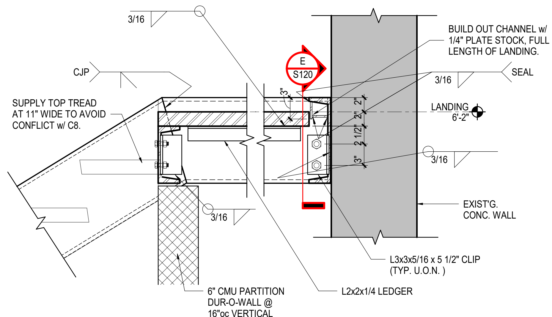
(D) STAIR LANDING LOW STRINGER CONN. 1 1/2" = 1'-0"
